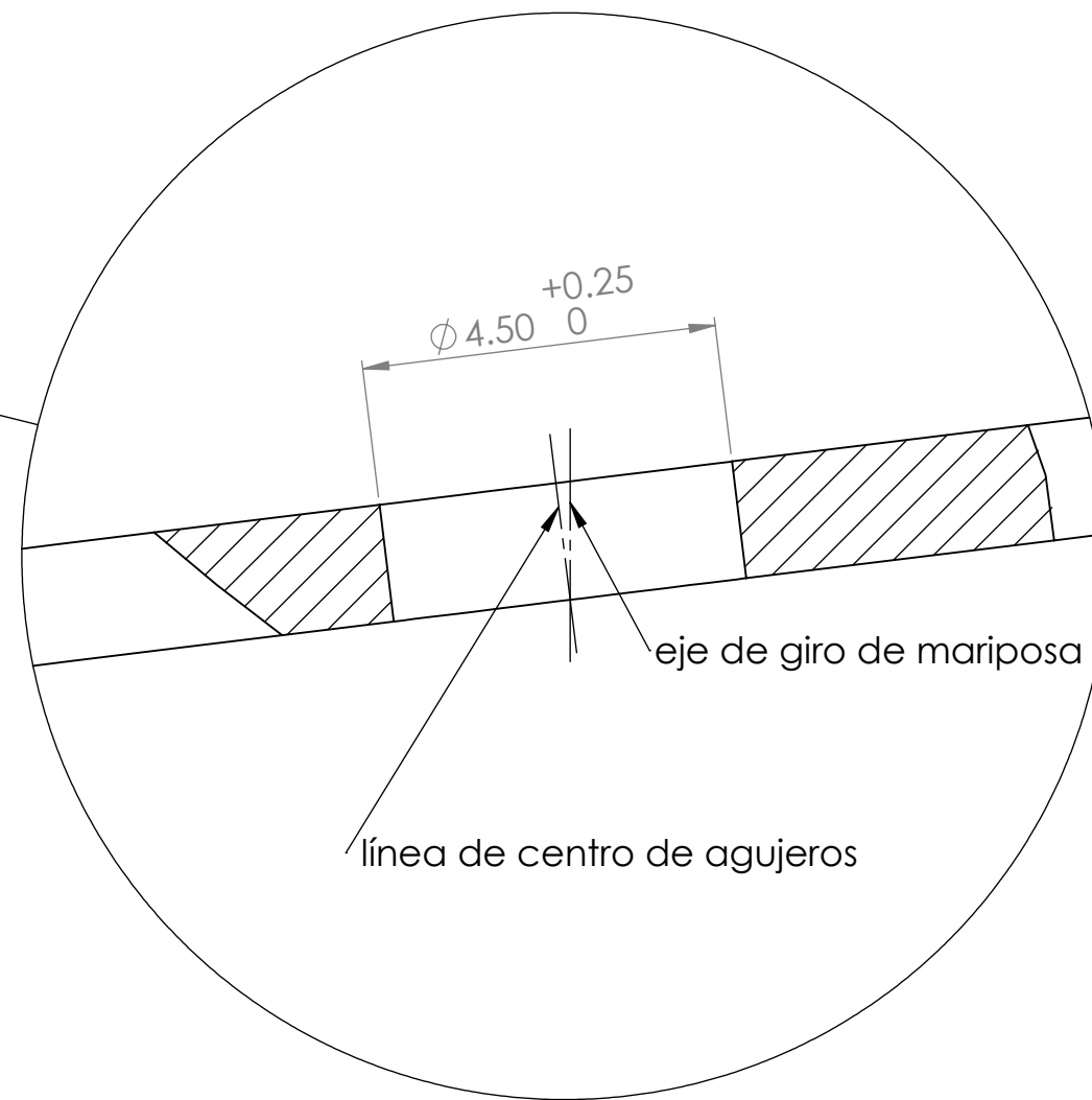
DETALLE A 10 : 1
